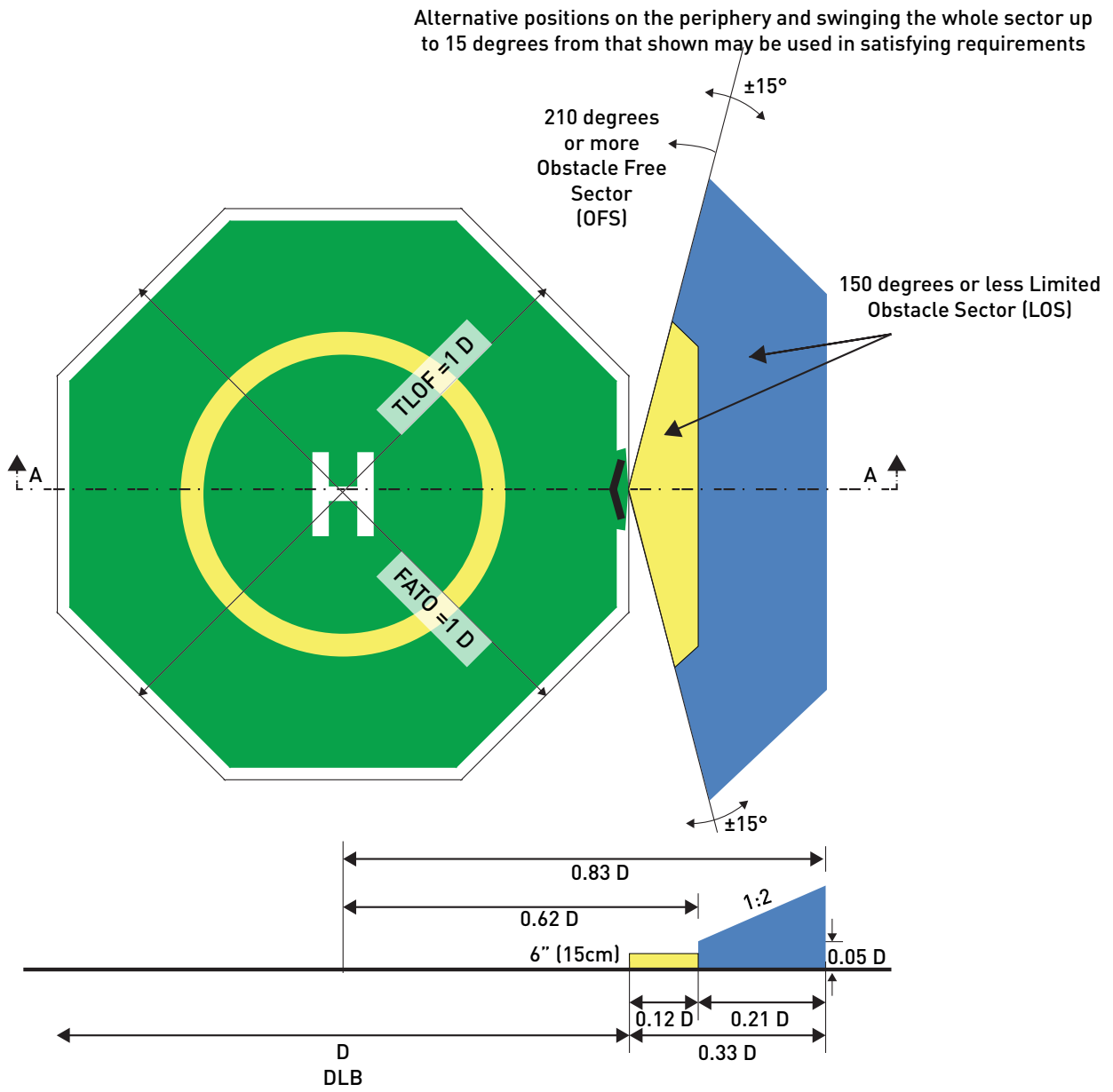
Section A-A
